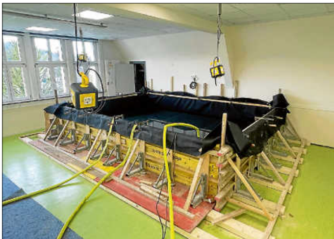
In der Werkrealschule wurde zur Tragfähigkeitsprüfung ein Wasserbecken aufgebaut. Foto: Stadt Hch
